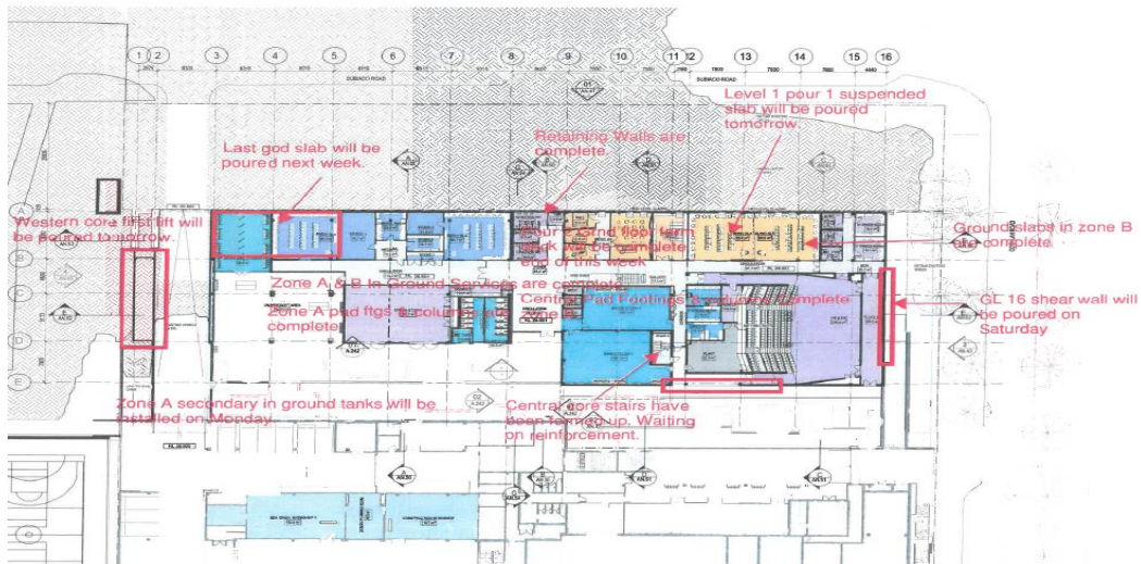
SETOUT PLAN - LG
